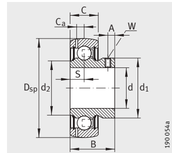
GAY..-NPP-B
