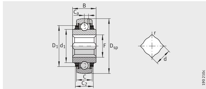
GVK..-KTT-B(-AH.), VK..-KTT-B(-AH.)
